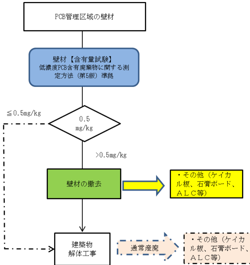
図 10-5 壁材・天板の解体撤去の流れ
