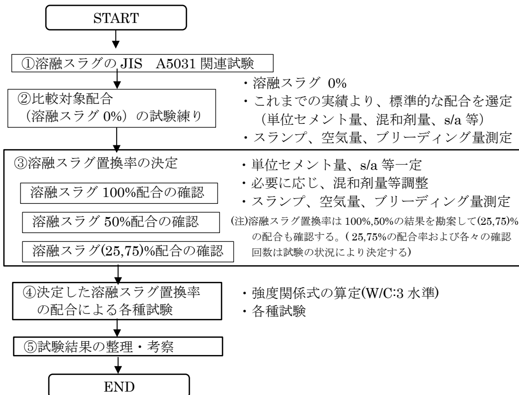
図-2 コンクリート骨材としての適用性確認試験フロー
