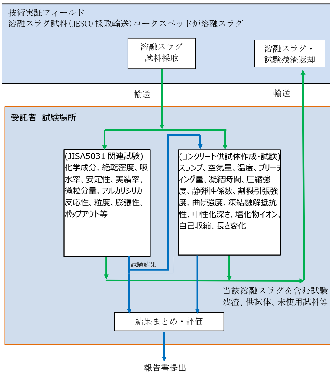
図-1 溶融スラグを骨材として使用したコンクリートの品質検討業務フロー
