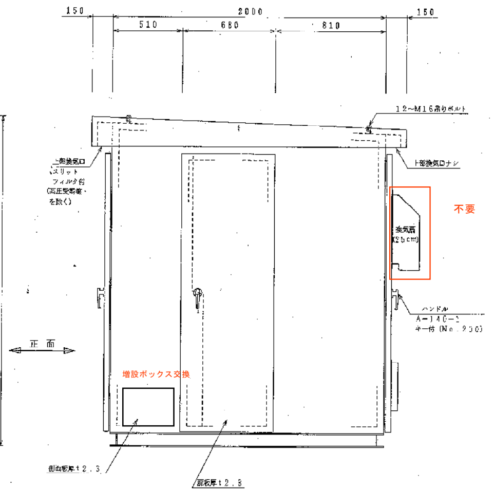
右側面図
