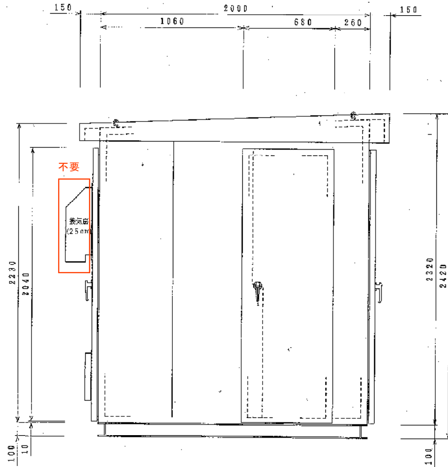
左側面図
