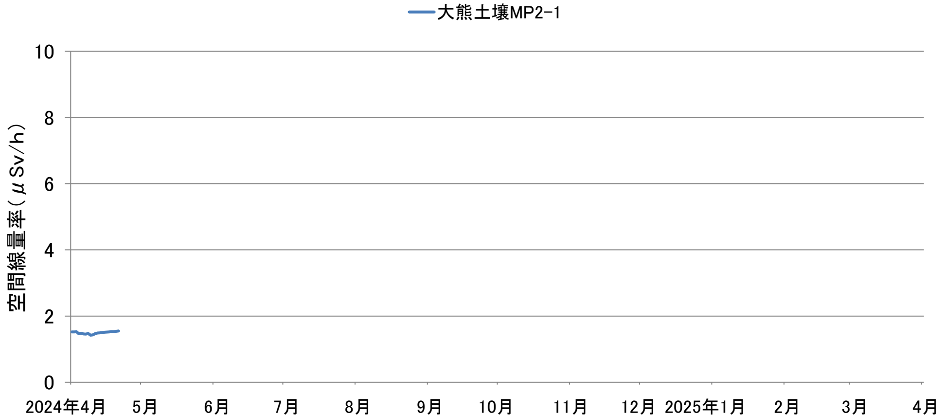
土壤貯蔵施設（大熊①工区）境界における空間線量率の推移（連続測定） （2024年4月1日～4月21日）
