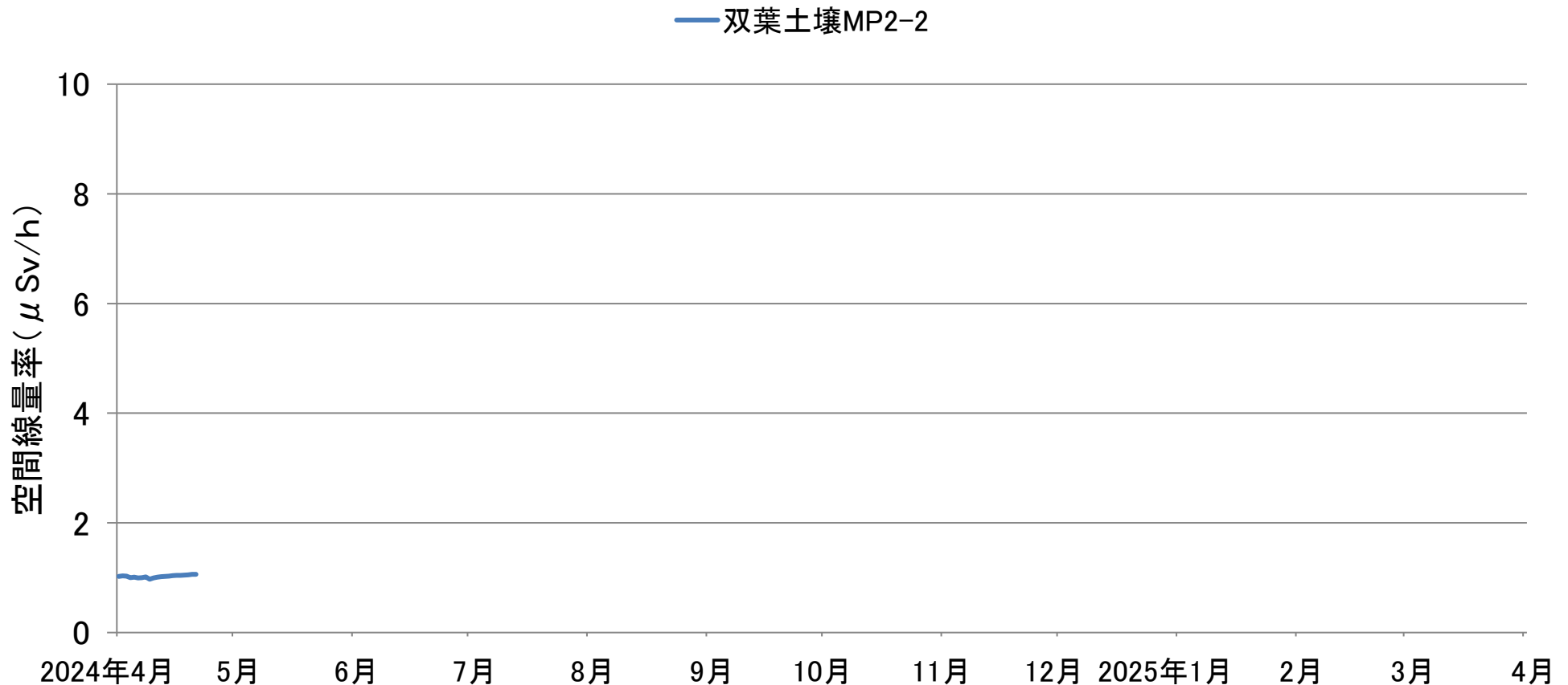
土壤貯蔵施設（双葉②工区）境界における空間線量率の推移（連続測定） （2024年4月1日～4月21日）
