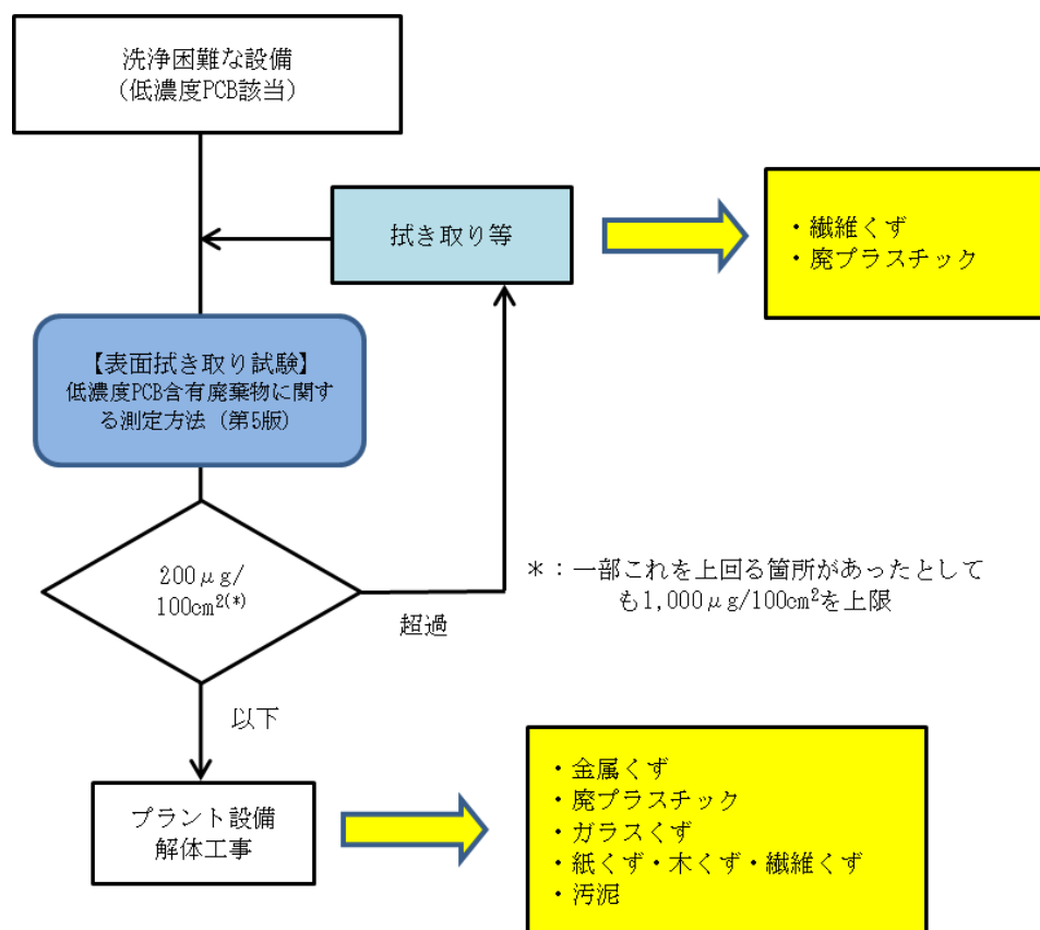
図 10-3 洗淨困難なプラント設備（高濃度 PCB 付着なし）の解体撤去の流れ
