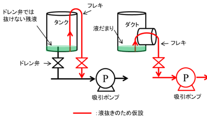
図2-1 吸引ポンプを用いたドレン弁、液だまりの洗浄
