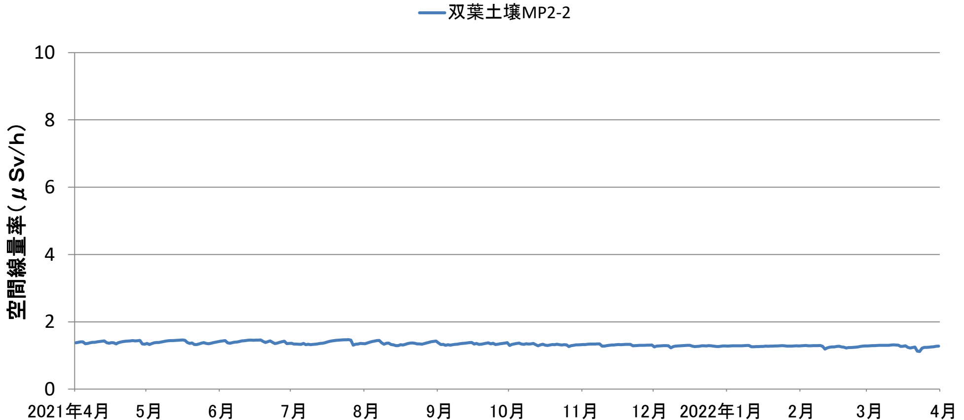
土壤貯蔵施設（双葉②工区）境界における空間線量率の推移（連続測定） （2021年4月1日～2022年3月31日）
