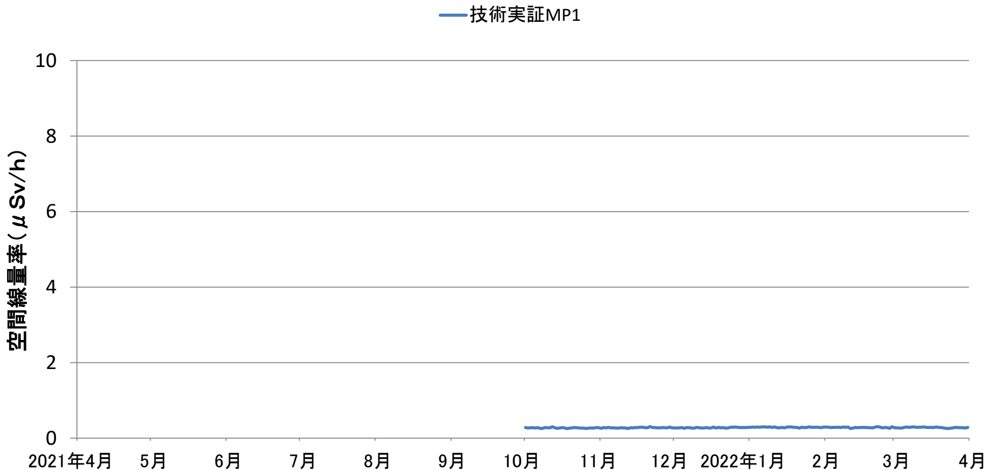
技術実証フィールド敷地内における空間線量率の推移(連続測定) (2021年4月1日～2022年3月31日)
