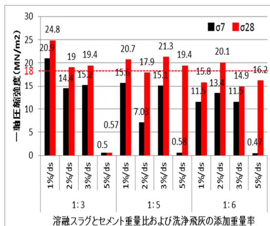
図 2-4 一軸圧縮強度試験の結果
