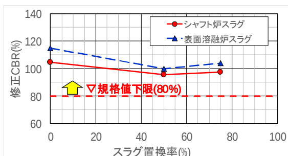
図 2-5 スラグ置換率と修正 CBR(95)
