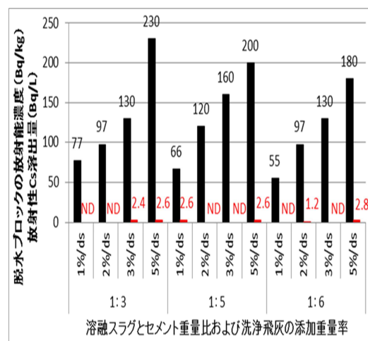
図 2-5 脱水固化体の放射性 Cs 濃度と放射性 Cs 溶出量
