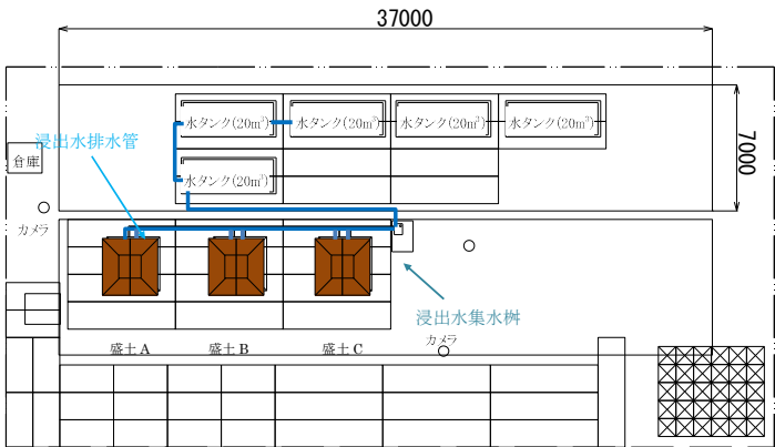
図 2-5 実証盛土配置図
