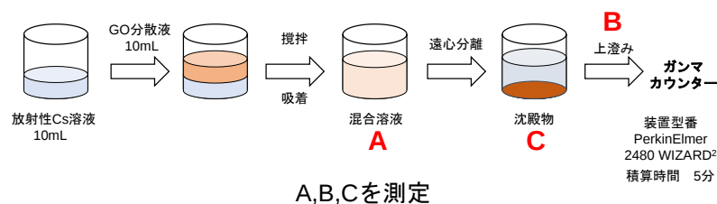
図3 放射性Cs吸着試験の操作手順
