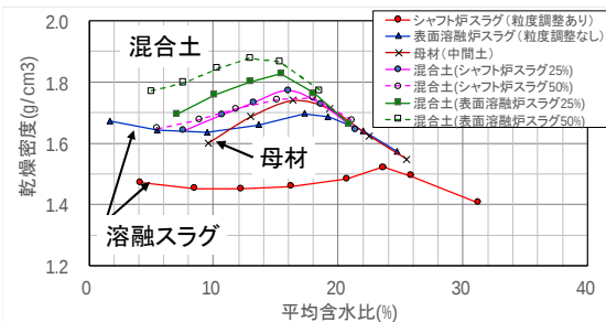
図 2-2 盛土試験で得られた締め固め曲線
