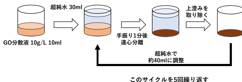
図4 GOの洗浄手順
