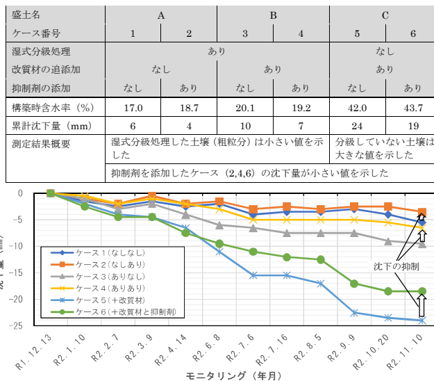
図 3-1 沈下量測定結果
