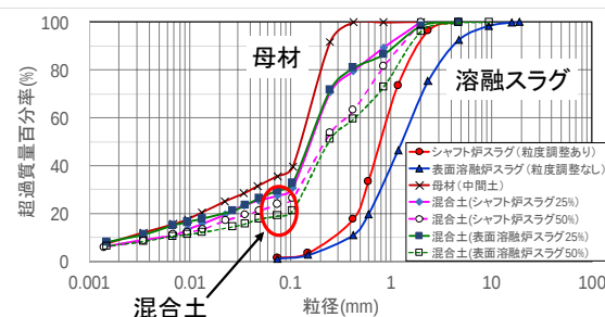
図 2-3 盛土材等の粒径加積曲線
