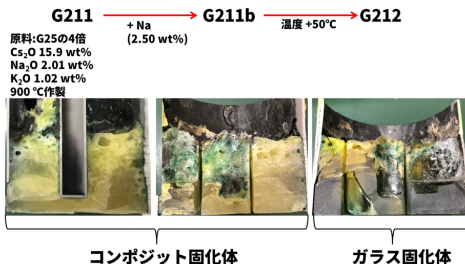
図 2-5 ウォータージェット法により切断した G211、G211b、G212 固化体
