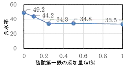
図 2-3 抑制剤添加量とふるい上残留物の含水比
