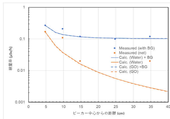
図 12 Cs-137 を含む GO 吸着残渣を入れたビーカー表面からの距離と線量率の測定値と計算値との比較結果
