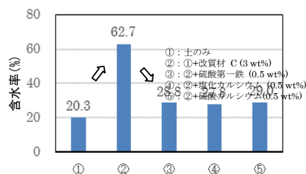
図 2-2 ふるい上残留物の含水率
