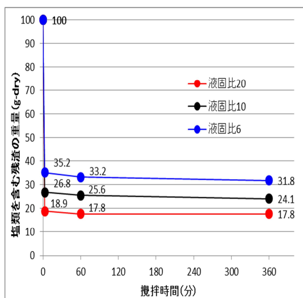
図 2-2 溶媒の液固比と攪拌時間の関係
