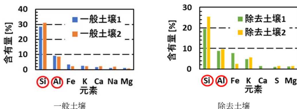
図 4-1 XRF による元素組成分析結果
