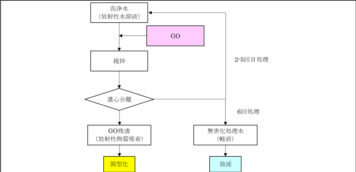
図 9 溶融飛灰洗浄水の処理フロー
