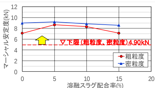
図 2-6 溶融スラグ配合率とマーシャル安定度
