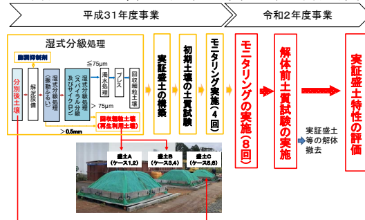
図 1 実証技術の概要
