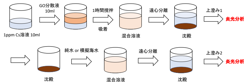
図 2 GO からの吸着した Cs の再溶出試験の手順
