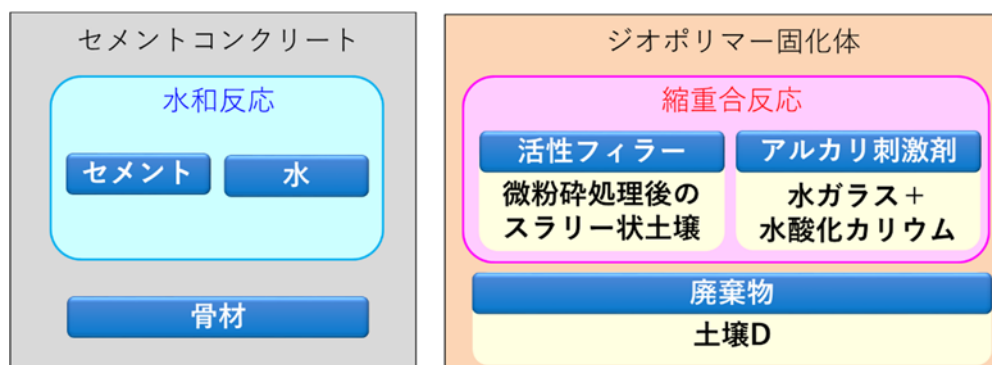
図 2-2 ジオポリマー技術の概略説明図
