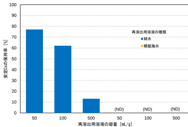
図6 再溶出試験用溶液下でのGOに吸着した安定Csの保持率
