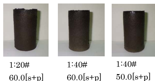
図 4-4 固化試験（除去土壌）
