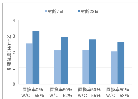
(引張強度)
