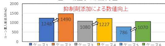
図 5 原位置コーン貫入試験
