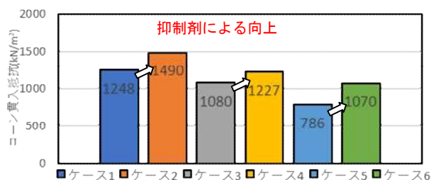
図 3-3 原位置コーン貫入試験結果
