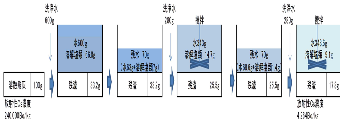
図 2-3 飛灰洗浄方法の模式図（溶融飛灰 100g 当り）
