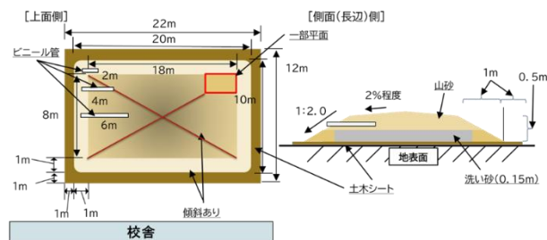
図 1 模擬施設完成図
