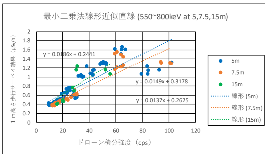
図 2-2 空間線量（1 m高さ）と積分強度（敷地境界除く）
