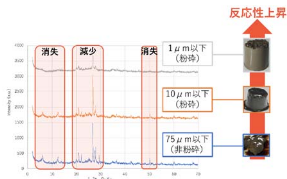
図 4-4 微粉碎によるジオポリマー固化への反応性上昇
