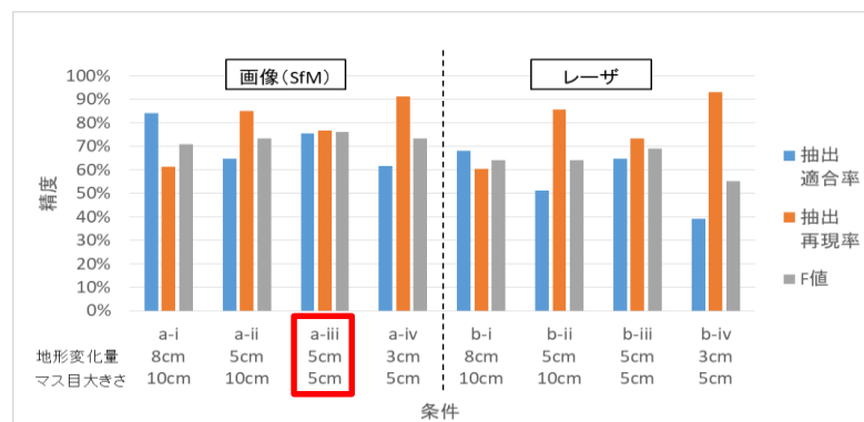
図 1-4 各条件における変状自動抽出の精度指標
