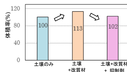
図 2-4 回収粗粒土壌の体積変化
