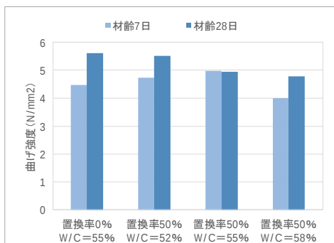
(曲げ強度)
