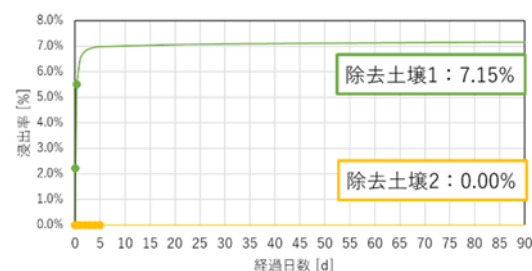
図 4-7 浸出試験結果（除去土壌）
