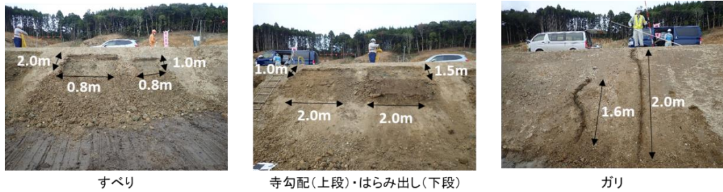
図 1-1 造作した模擬変状例の写真
