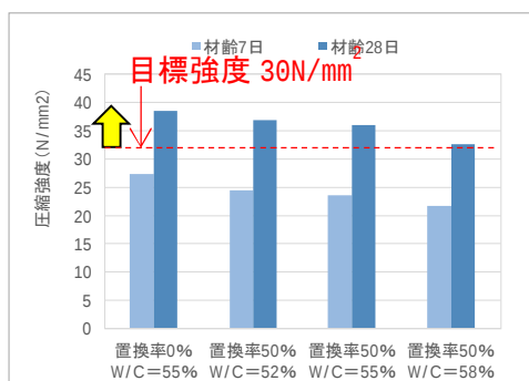
(圧縮強度)
