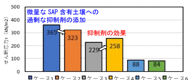
図 3-4 一面せん断試験（攪乱）結果
