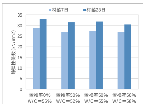
(静弾性係数)
