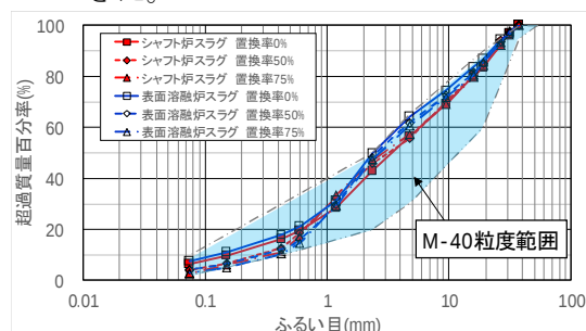
図 2-4 路盤材試験供試体の粒径加積曲線
