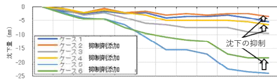
図 3 実証盛土の沈下量測定
