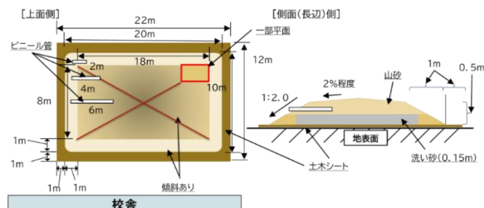
図 3-2 模擬施設完成図
