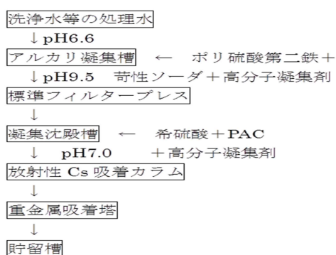
図 2-7 洗浄水等の処理フロー
