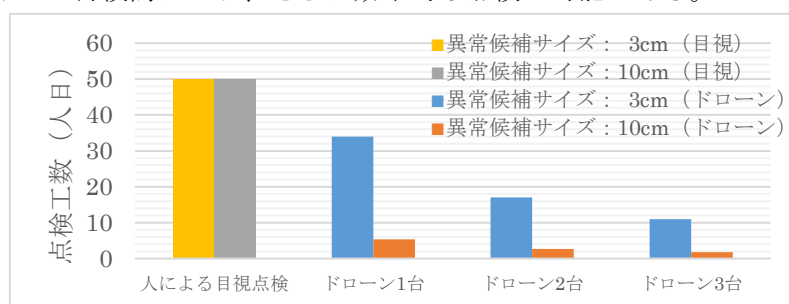
図 3-15 ドローン台数・異常候補サイズからみる点検工数
