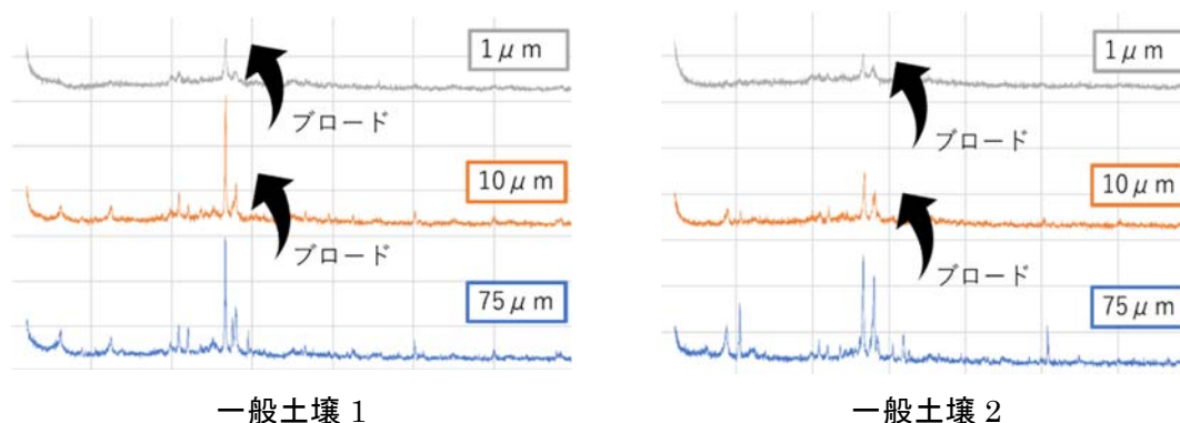
図 4-2 微粉碎試験のXRD変化（一般土壤）
