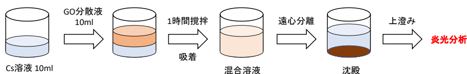
図 1 GO 吸着性能評価のための実験操作
