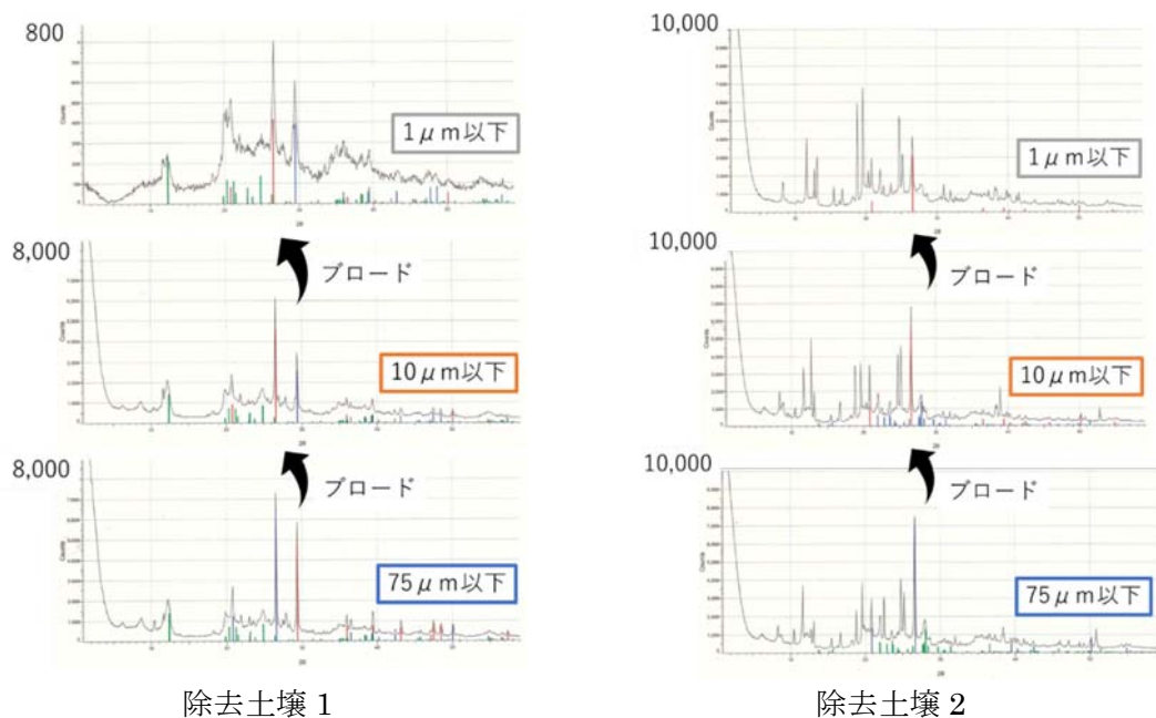
図 4-3 微粉碎試験の XRD 変化（除去土壌）
