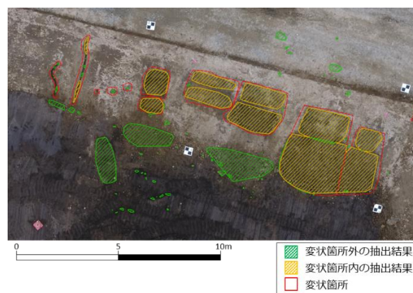
図 1-5 条件 a-iii（画像、地形変化量 5cm、マス目大きさ 5cm）における変状自動抽出結果
