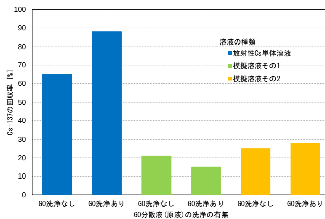
図7 洗浄あり／なしのGOによる放射性Csの回収率の比較
