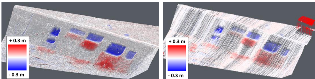
図 1-2 二時期点群の差分量の可視化例（左；画像 右：レーザ）
