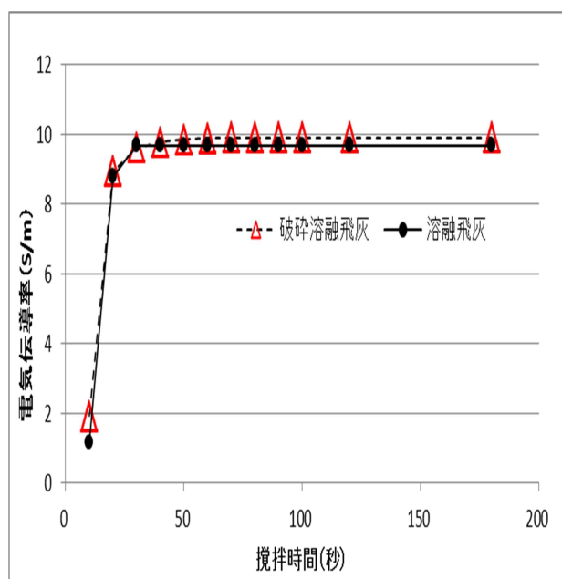
図 2-1 事前破碎の要否の確認
