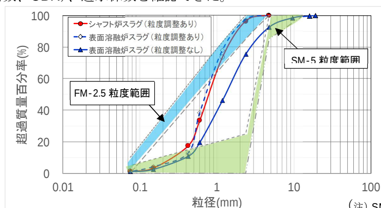
図 2-1 熔融スラグの粒径加積曲線
