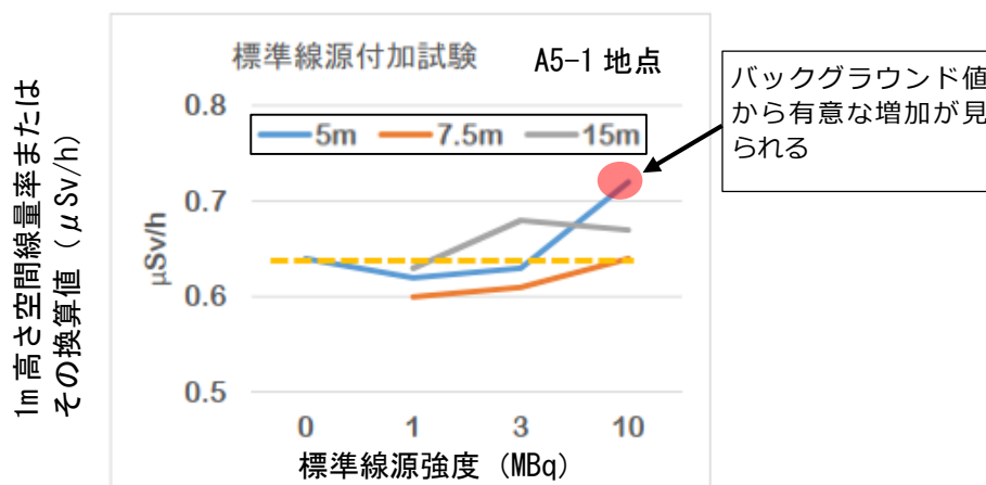
図 2-4 A 区域 A5-1 での空間線量率換算値
