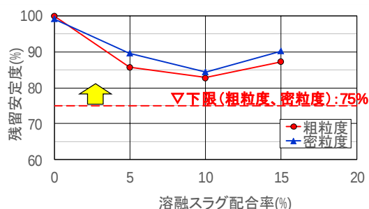
図 2-7 溶融スラグ配合率と残留率
