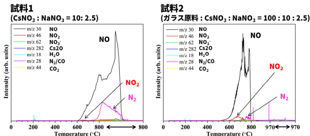
図 2-2 試料 1 および 2 の加熱時におけるガス発生挙動
