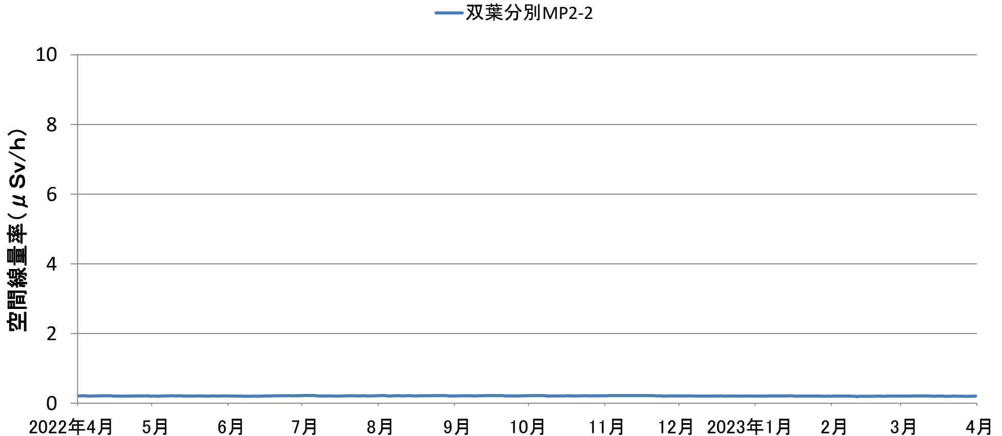
受入・分別施設(双葉②工区)境界における空間線量率の推移(連続測定) (2022年4月1日 ~ 2023年3月31日)
