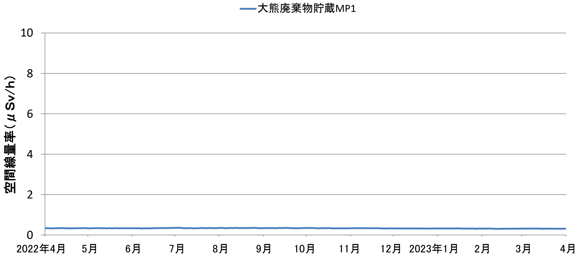
廃棄物貯蔵施設（大熊1工区）境界における空間線量率の推移（連続測定） （2022年4月1日～2023年3月31日）
