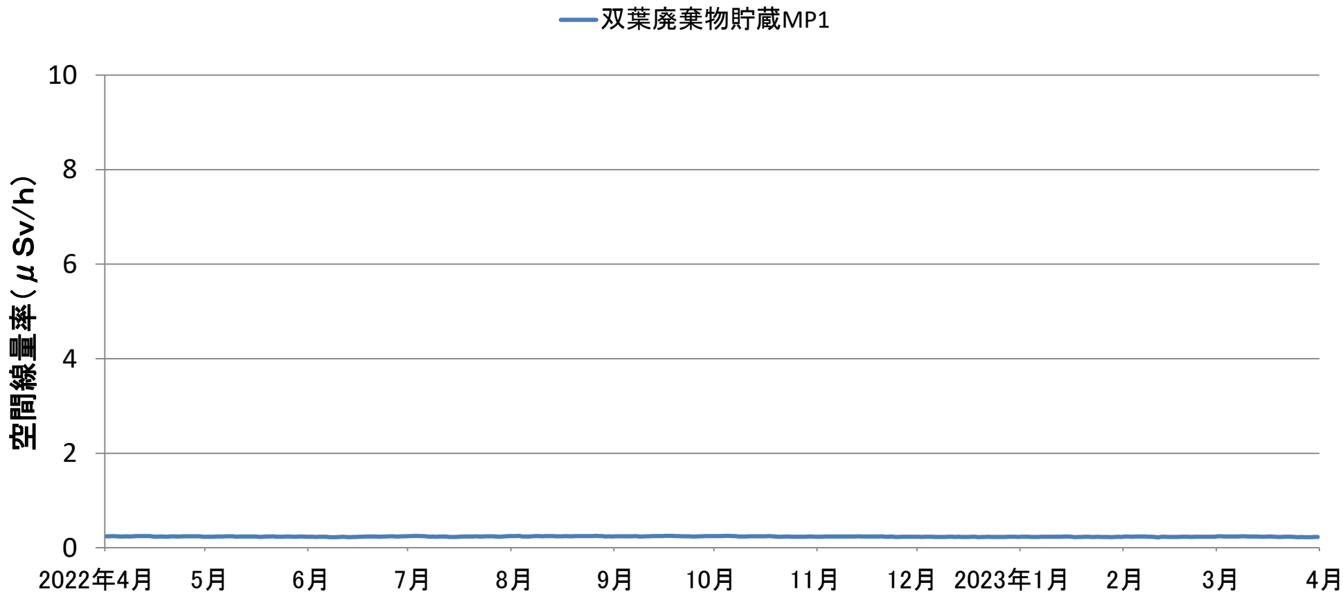
廃棄物貯蔵施設（双葉1工区）境界における空間線量率の推移（連続測定） （2022年4月1日～2023年3月31日）
