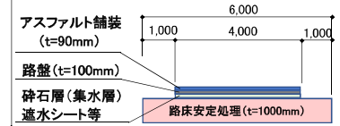
図4 舗装道路断面図
