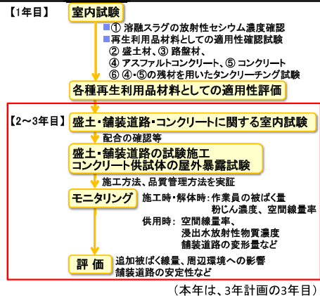
図1 実証事業のフロー
