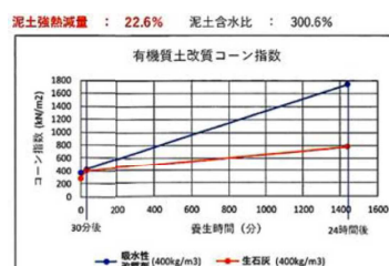
図3 吸水性固化材による有機汚泥改質試験例
