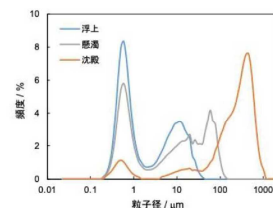
図5 加圧浮上処理物の粒径分布（ラボ試験）
