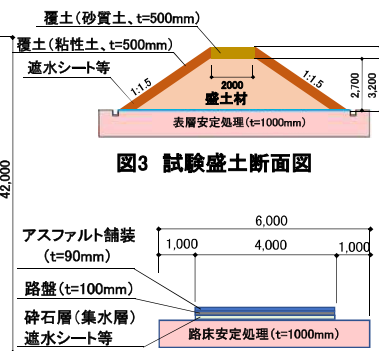
図4 舗装道路断面図
