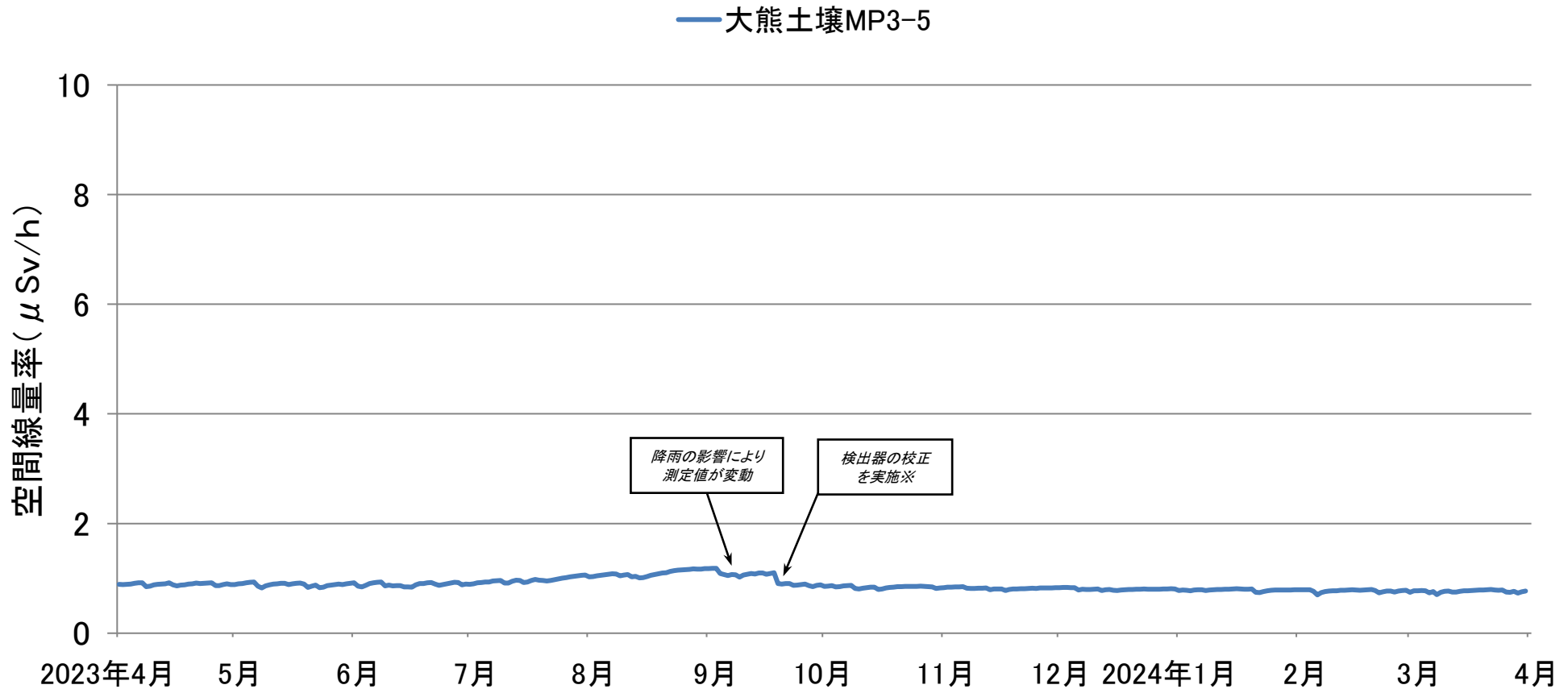
土壤貯蔵施設（大熊⑤工区）境界における空間線量率の推移（連続測定） （2023年4月1日～2024年3月31日）
