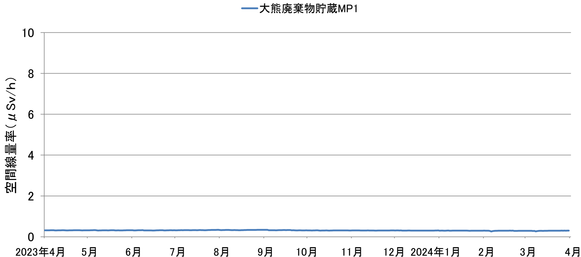
廃棄物貯蔵施設（大熊1工区）境界における空間線量率の推移（連続測定） （2023年4月1日～2024年3月31日）
