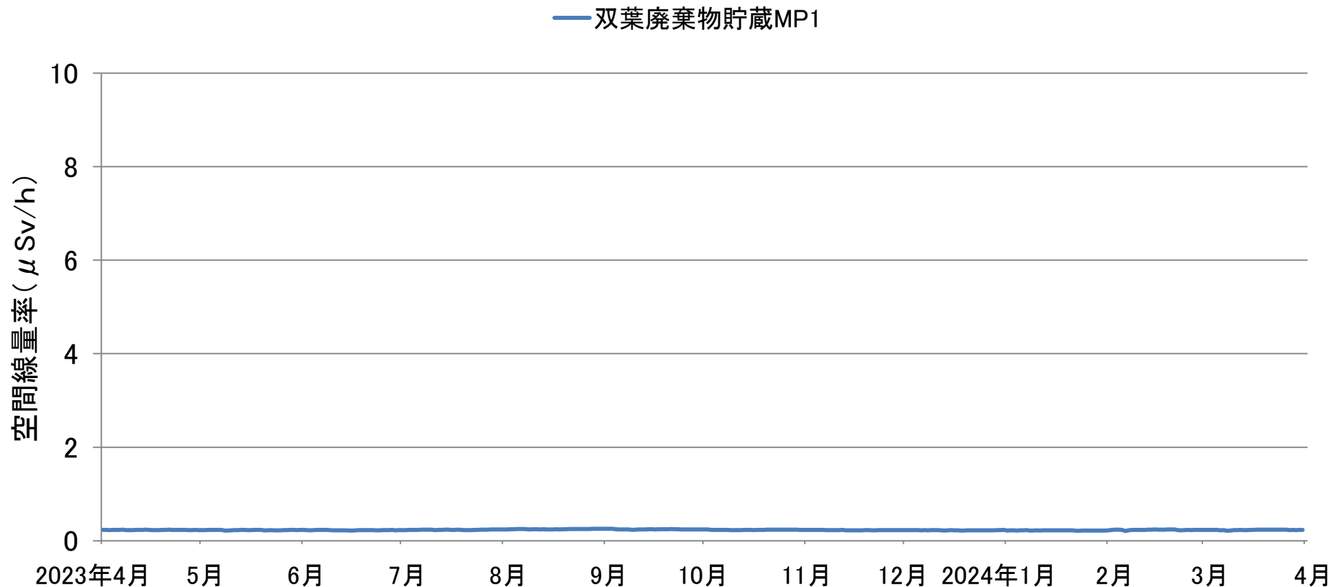
廃棄物貯蔵施設（双葉1工区）境界における空間線量率の推移（連続測定） （2023年4月1日～2024年3月31日）
