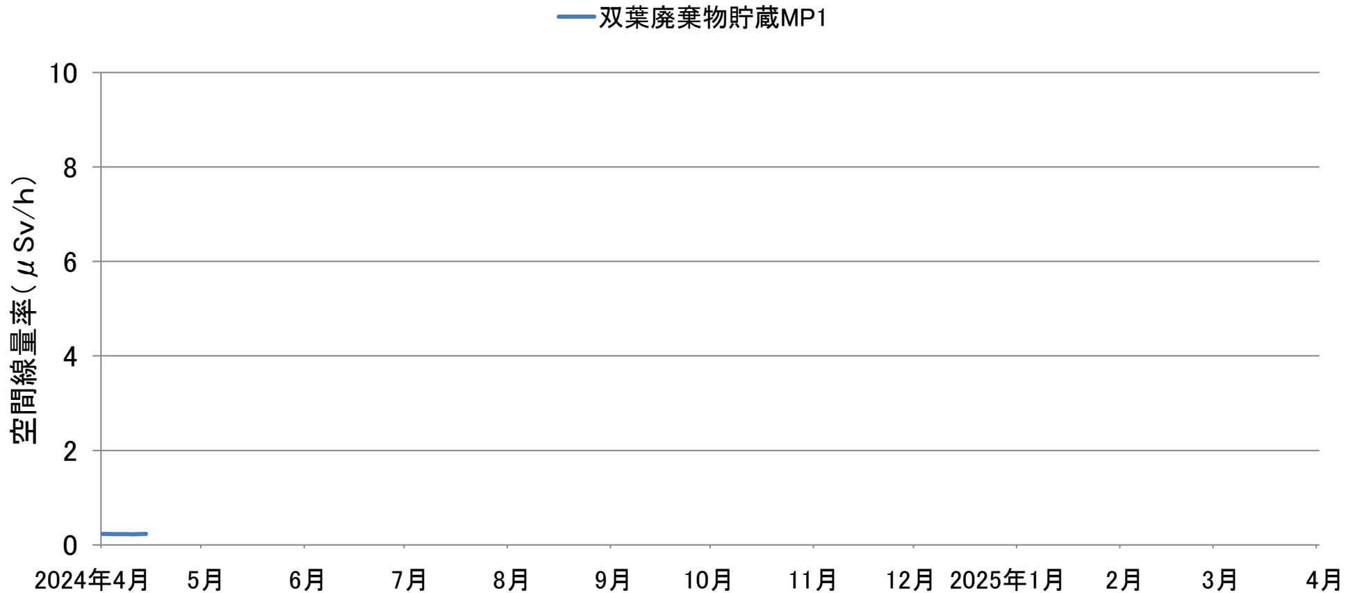
廃棄物貯蔵施設（双葉1工区）境界における空間線量率の推移（連続測定） （2024年4月1日～4月14日）
