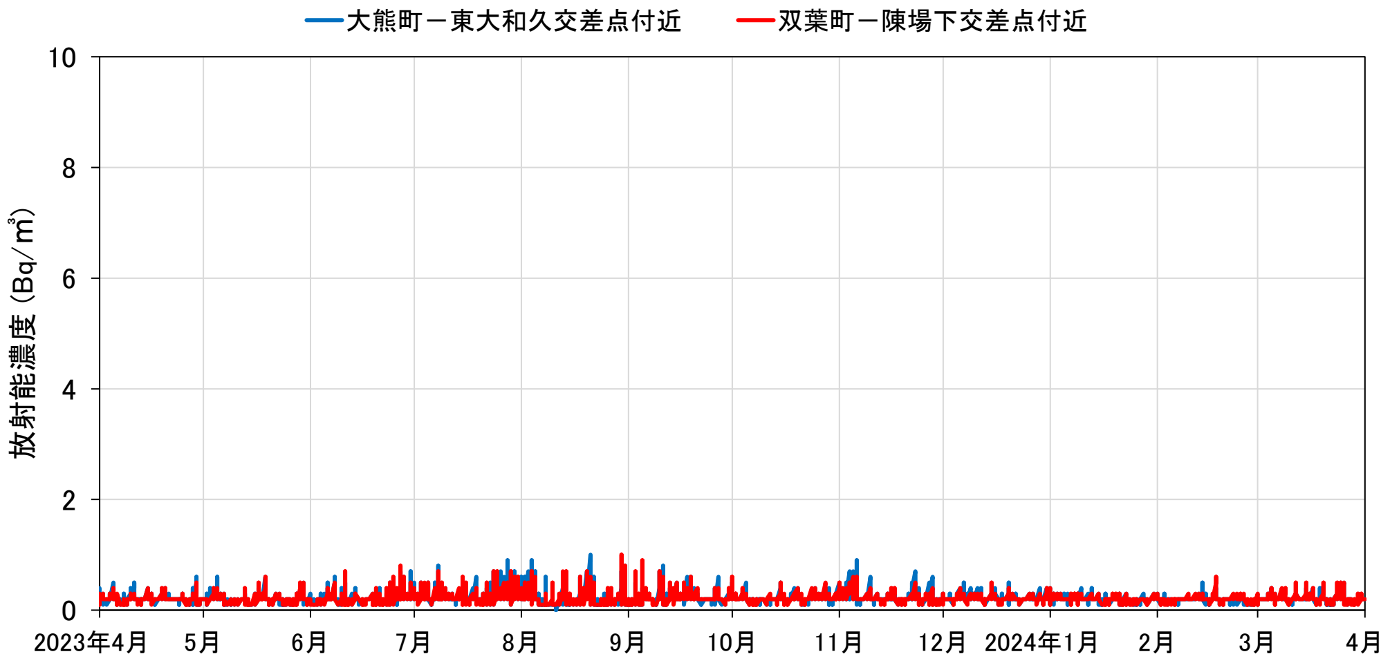
中間貯蔵施設区域境界における大気中のβ線の放射能濃度(連続測定) (2023年4月1日～2024年3月31日)
