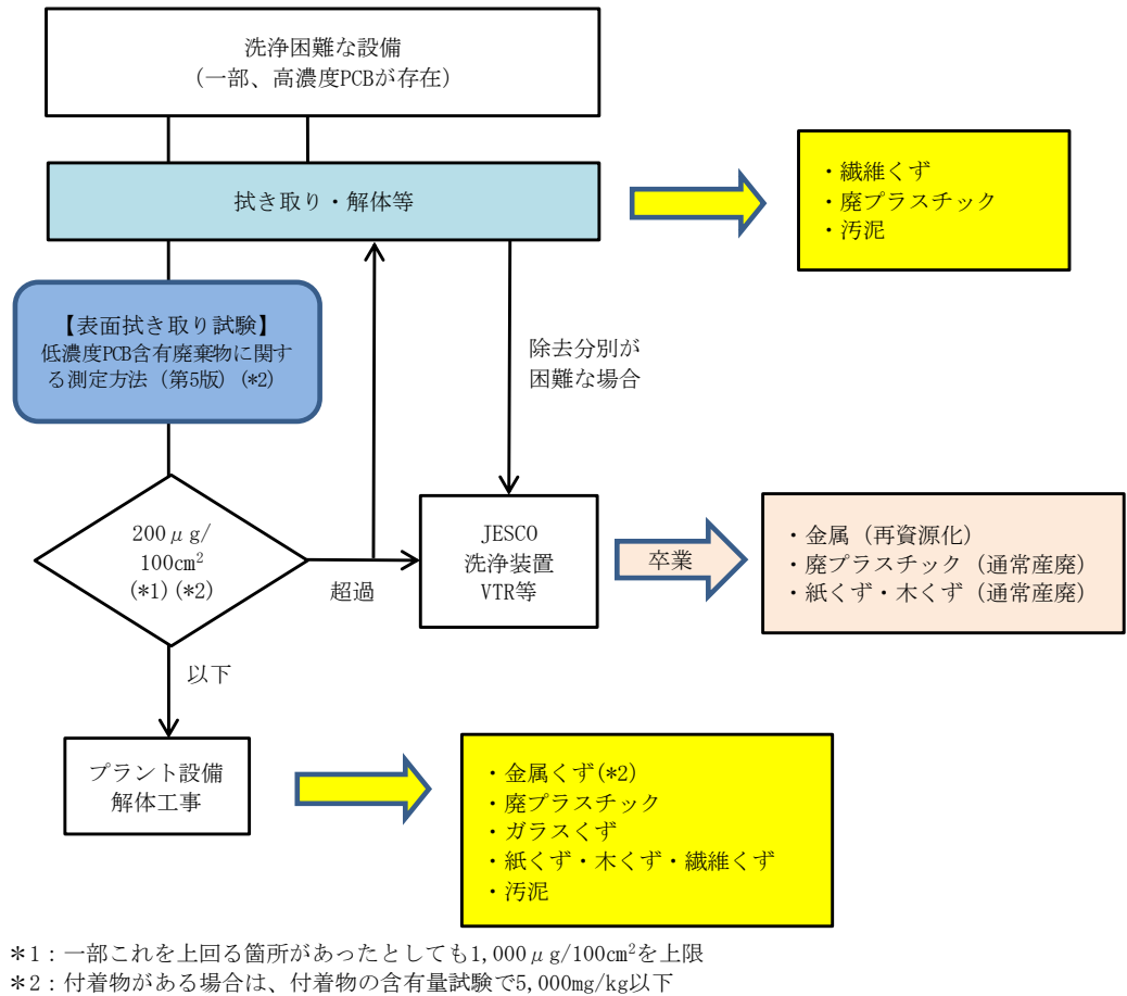
図 10-2 洗浄困難なプラント設備（一部高濃度 PCB 付着）の解体撤去の流れ
