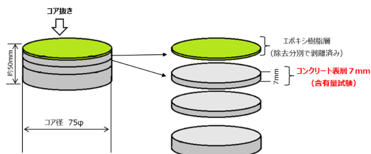
図 10-8 コンクリート表層のサンプリング方法
