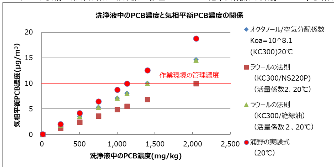
図 6-2 洗剤液中の PCB 濃度と気相平衡 PCB 濃度の関係
