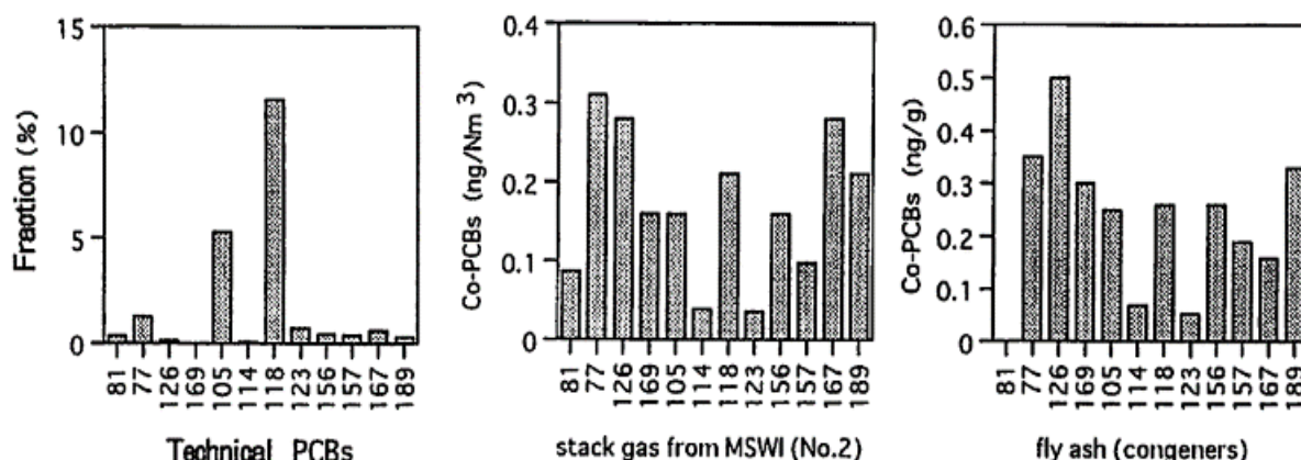
図 2-8 PCB 製品と燃焼排ガスと飛灰の Co-PCB 異性体分布
