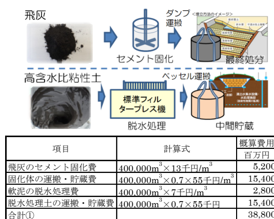
図 4-1 従来技術の概念と概算費用
