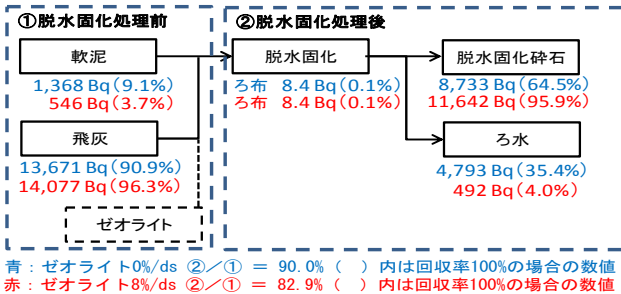
図 3-1 放射能収支のフロー（平均）
