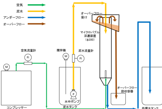
図 3-3 MBF 試験装置概要
