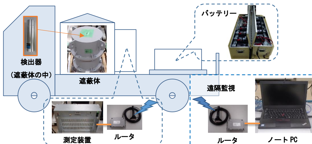
図 2-2 試験装置
