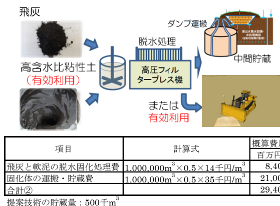
図 4-2 提案技術の概念と概算費用
