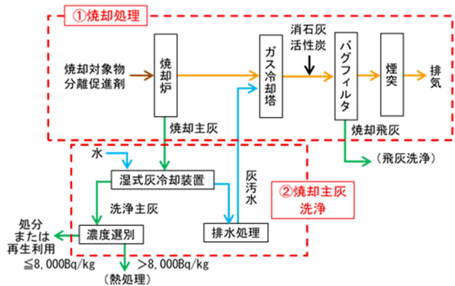
図 1 放射性 Cs 分離システム
