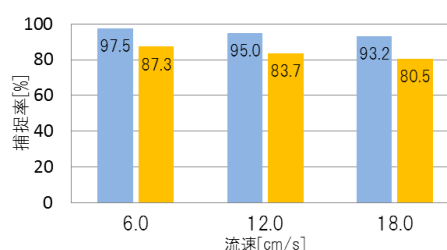
図 4-2 捕捉率試験結果 (左: 20 \mu\text{m} 未満、右: 20~75 \mu\text{m} )
