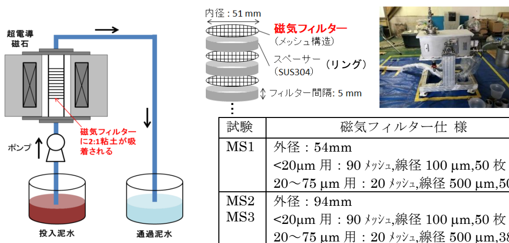
図 3-2 MS 試験装置概要
