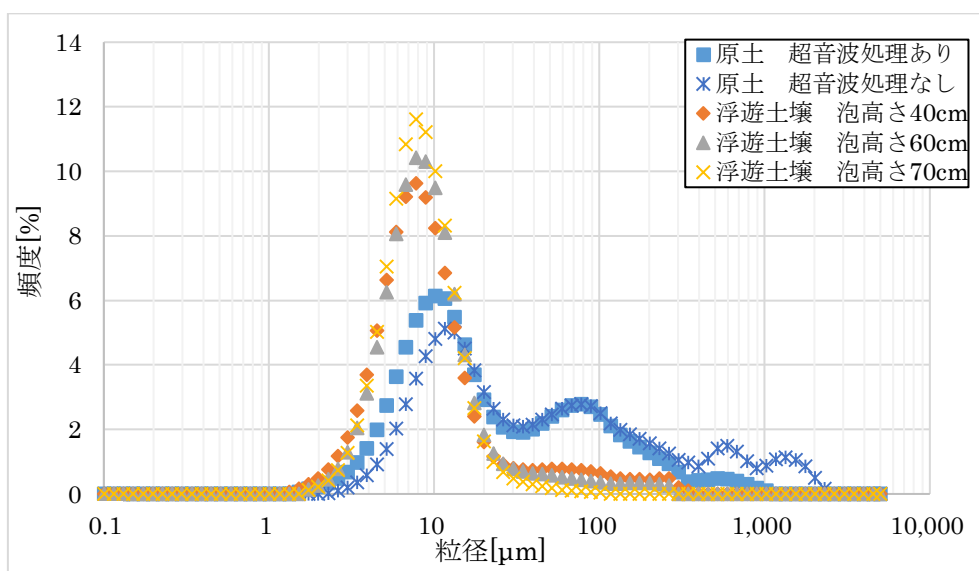
図 3-2 土壌 No.8A の粒子径分布
