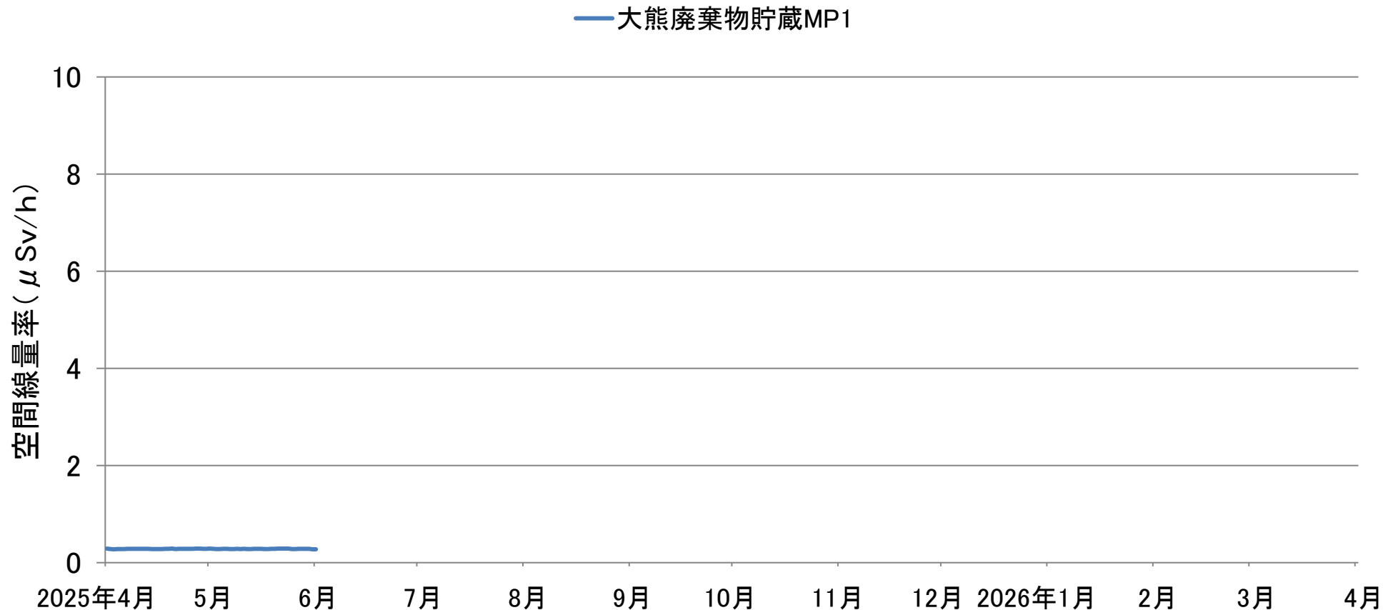
廃棄物貯蔵施設（大熊1工区）境界における空間線量率の推移（連続測定） （2025年4月1日～6月1日）
