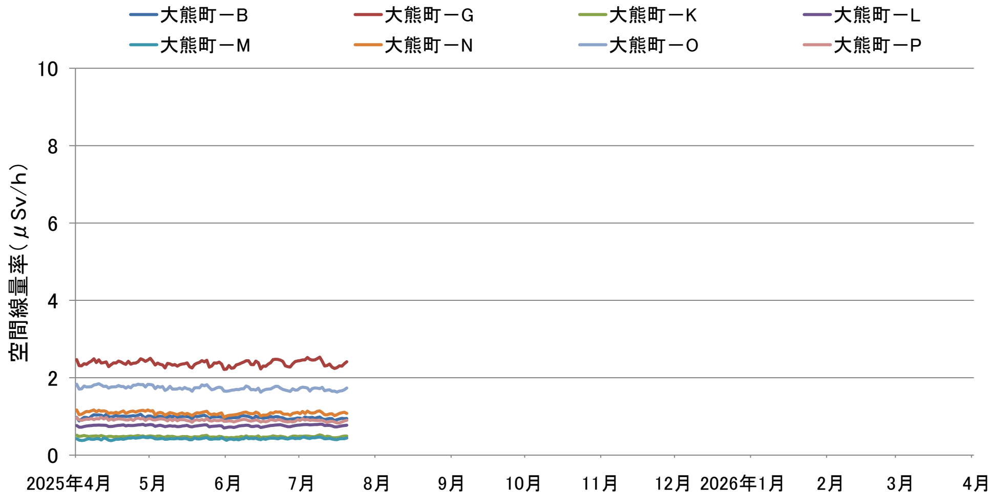
保管場等境界における空間線量率の推移(連続測定) (2025年4月1日～7月20日)
