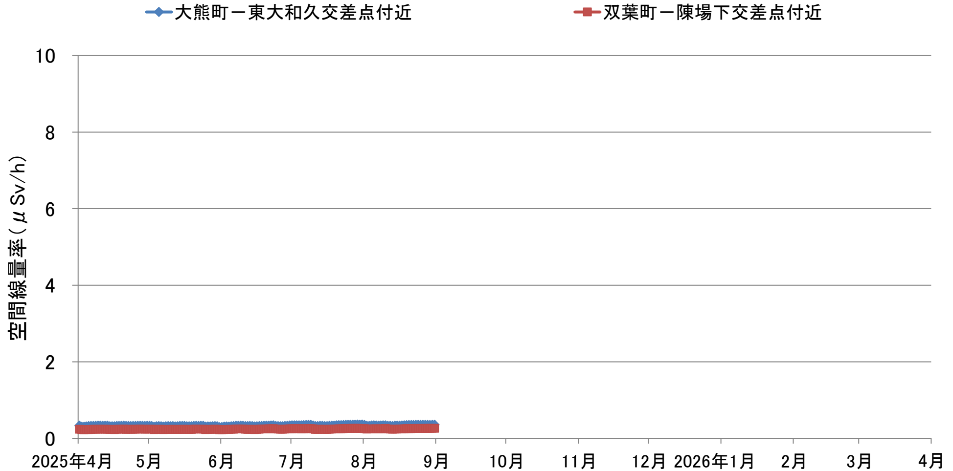
中間貯蔵施設区域境界における空間線量率の推移(連続測定) (2025年4月1日～8月31日)
