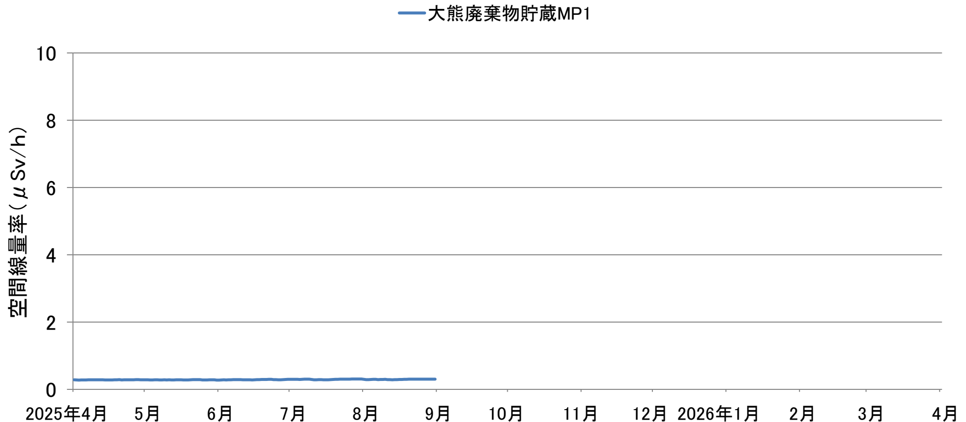
廃棄物貯蔵施設（大熊1工区）境界における空間線量率の推移（連続測定） （2025年4月1日～8月31日）
