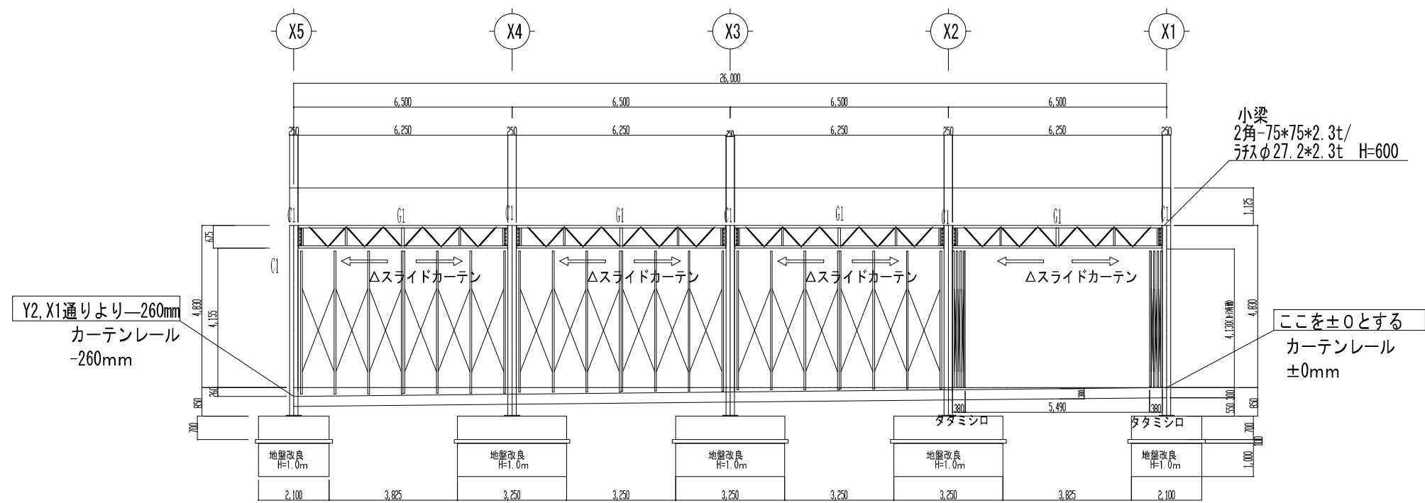
Y2通り 軸組図
