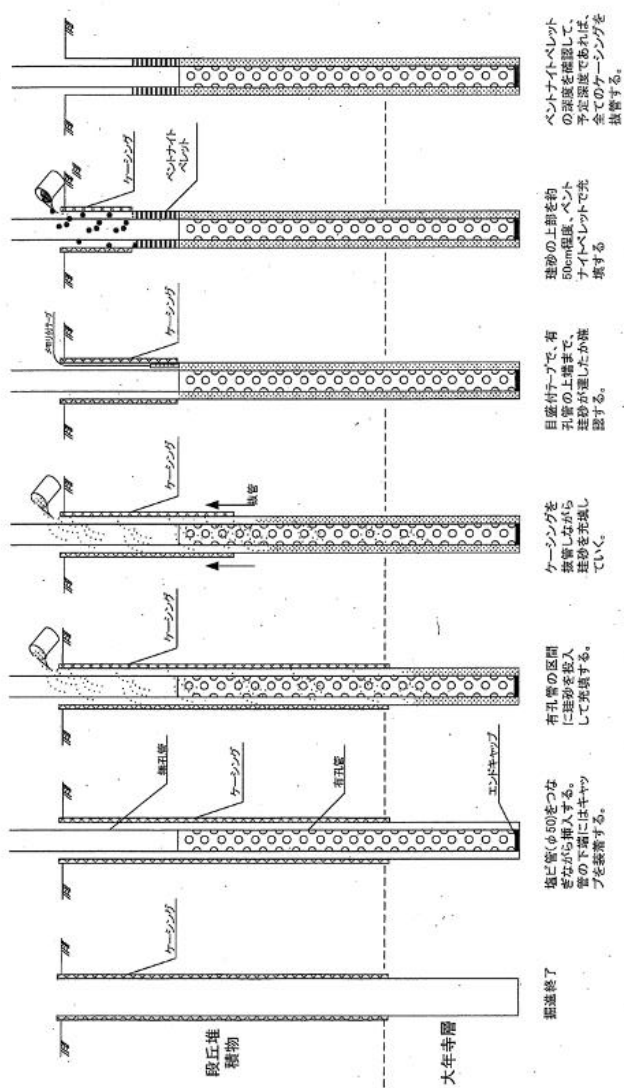
図 地下水観測井の設置手順 (その1)
