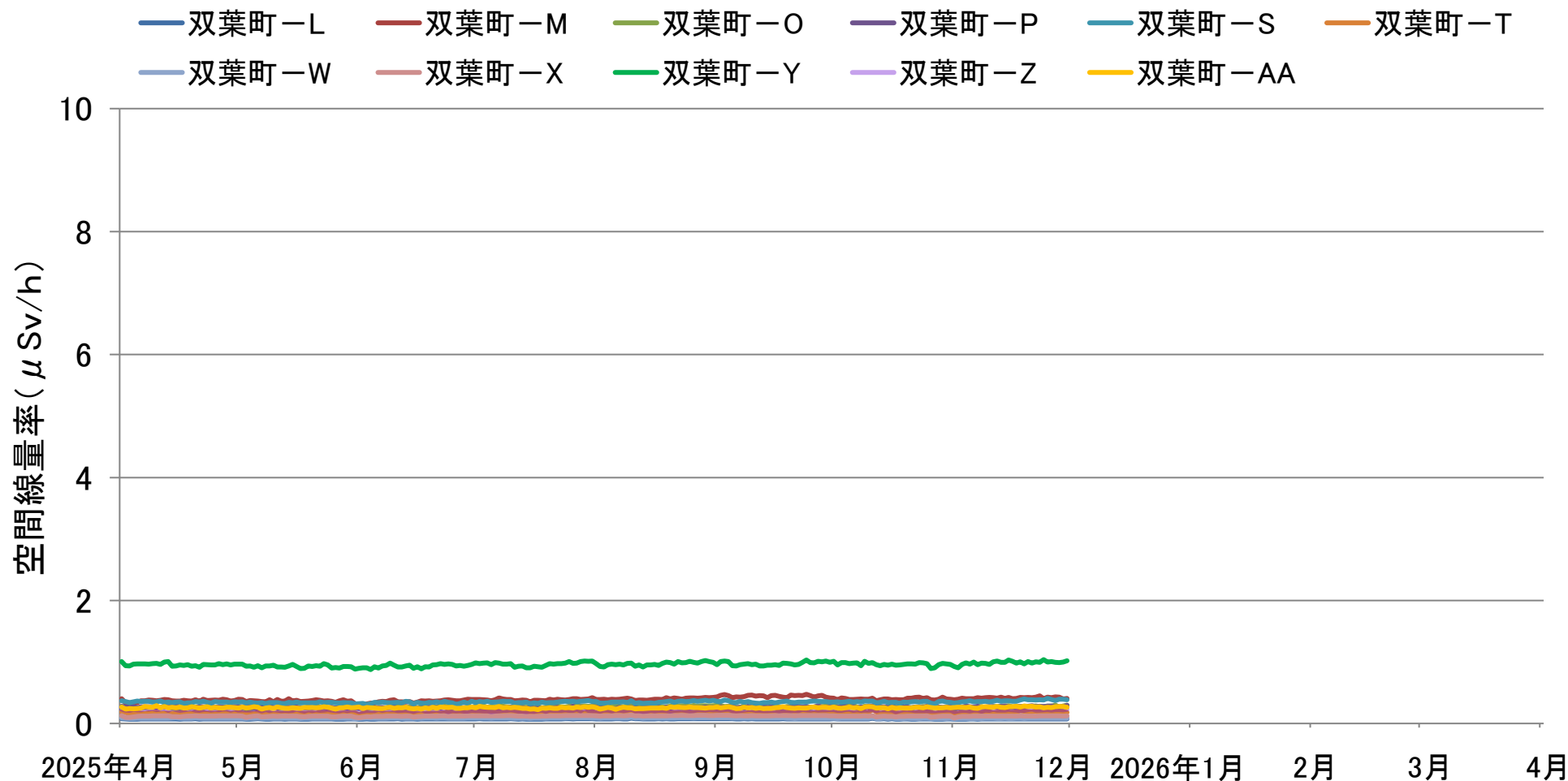
保管場等境界における空間線量率の推移(連続測定) (2025年4月1日 ~ 11月30日)
