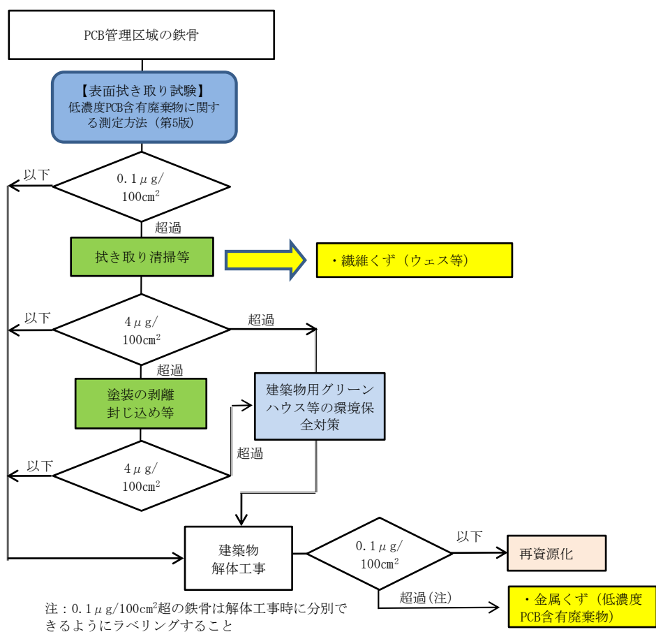
10-6 鉄骨の解体撤去の流れ
