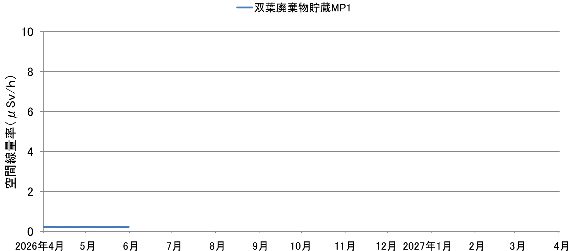
廃棄物貯蔵施設（双葉1工区）境界における空間線量率の推移（連続測定） （2026年4月1日～5月31日）
