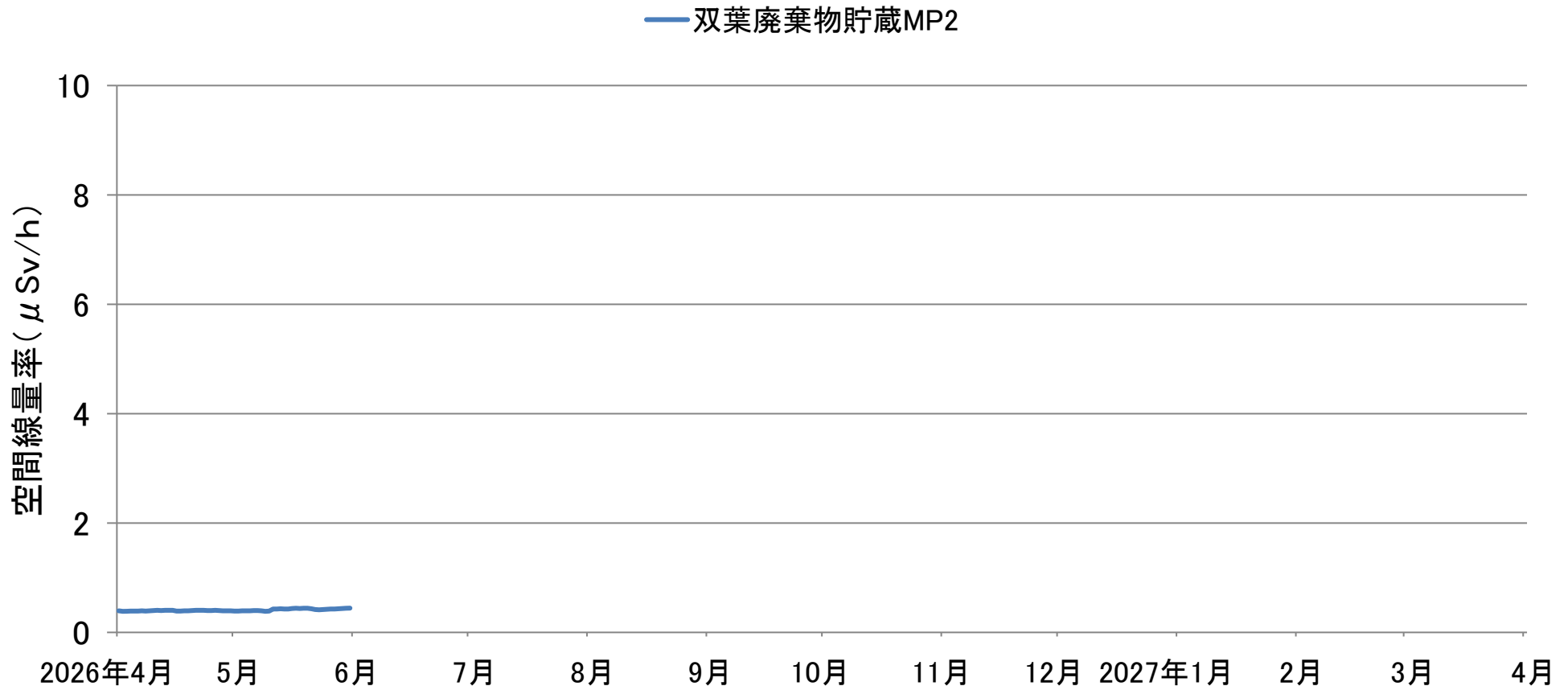
廃棄物貯蔵施設（双葉2工区）境界における空間線量率の推移（連続測定） （2026年4月1日～5月31日）
