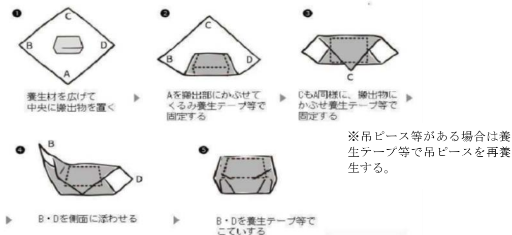
図 10-2 設備本体・盤等（自由液がないもの）の荷姿
