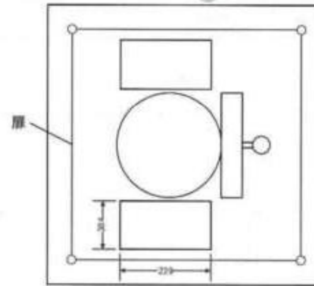
平面図
