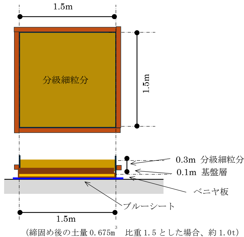
図－2 型枠設置イメージ
