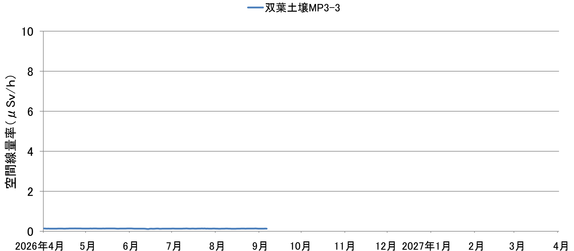
土壌貯蔵施設（双葉③工区）境界における空間線量率の推移（連続測定） （2026年4月1日～9月6日）
