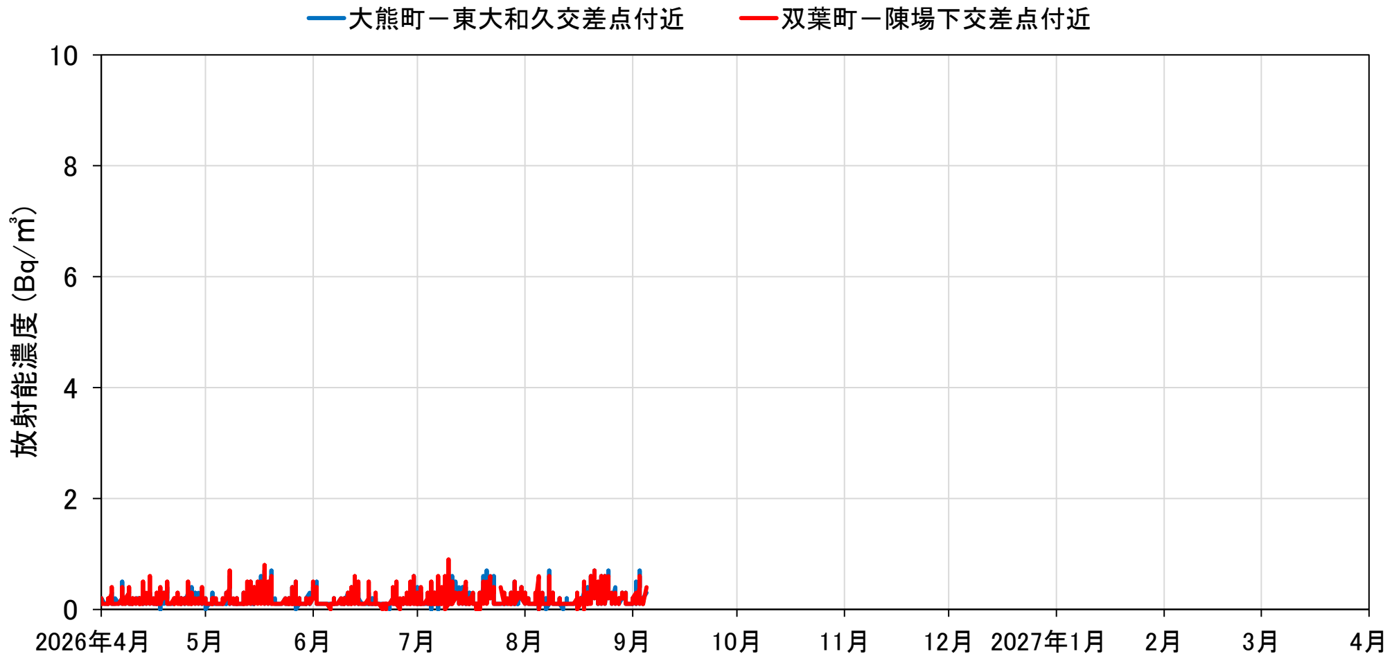
中間貯蔵施設区域境界における大気中の \beta 線の放射能濃度(連続測定) (2026年4月1日～9月4日)
