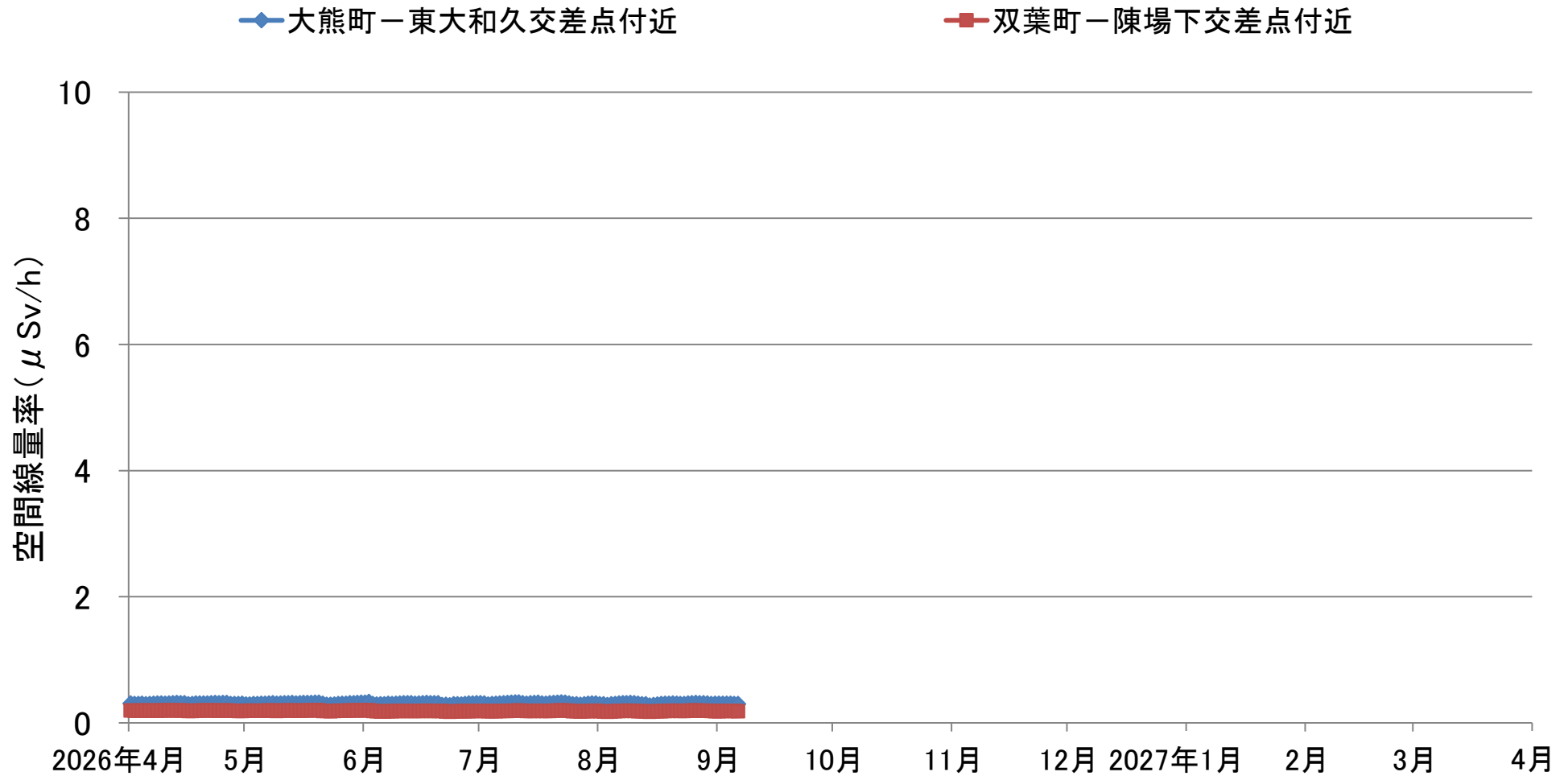
中間貯蔵施設区域境界における空間線量率の推移(連続測定) (2026年4月1日 ～ 9月6日)
