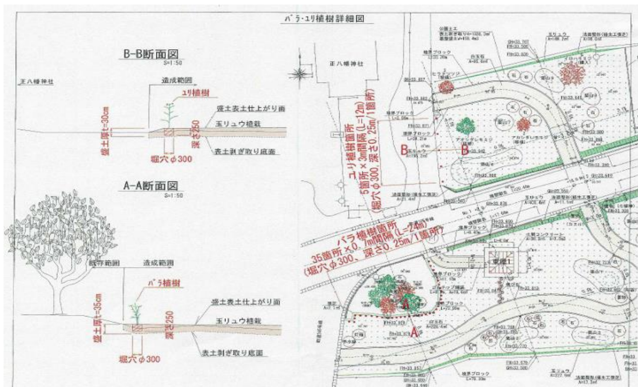
双葉町 正八幡神社周辺整備箇所（バラ・ユリ植樹詳細図）
