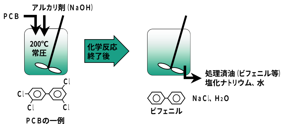
図 6.2-7 PCB分解方法概念図
