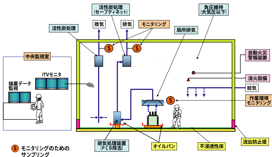
図 6.3-3 安全対策概念図
