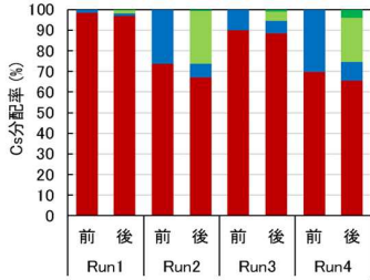
図5 洗浄前後のCsの挙動
