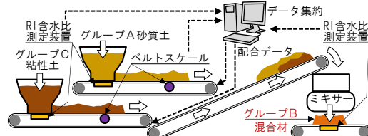
図2 試験装置のイメージ
