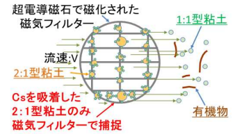
図1 MSの原理
