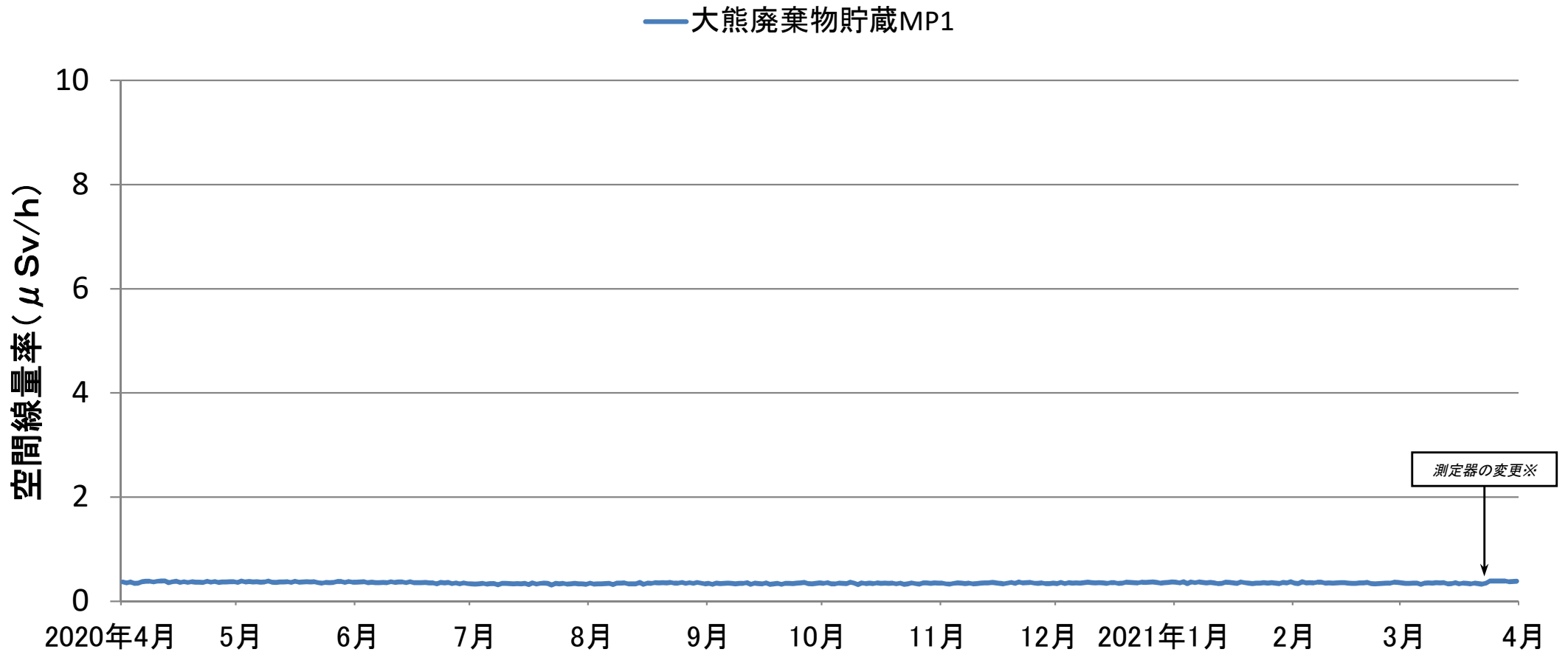
廃棄物貯蔵施設（大熊1工区）における空間線量率の推移（連続測定） （2020年4月1日～2021年3月31日）
